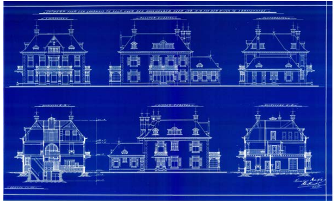
Bouwtekening Villa Arnhorst, 1912
